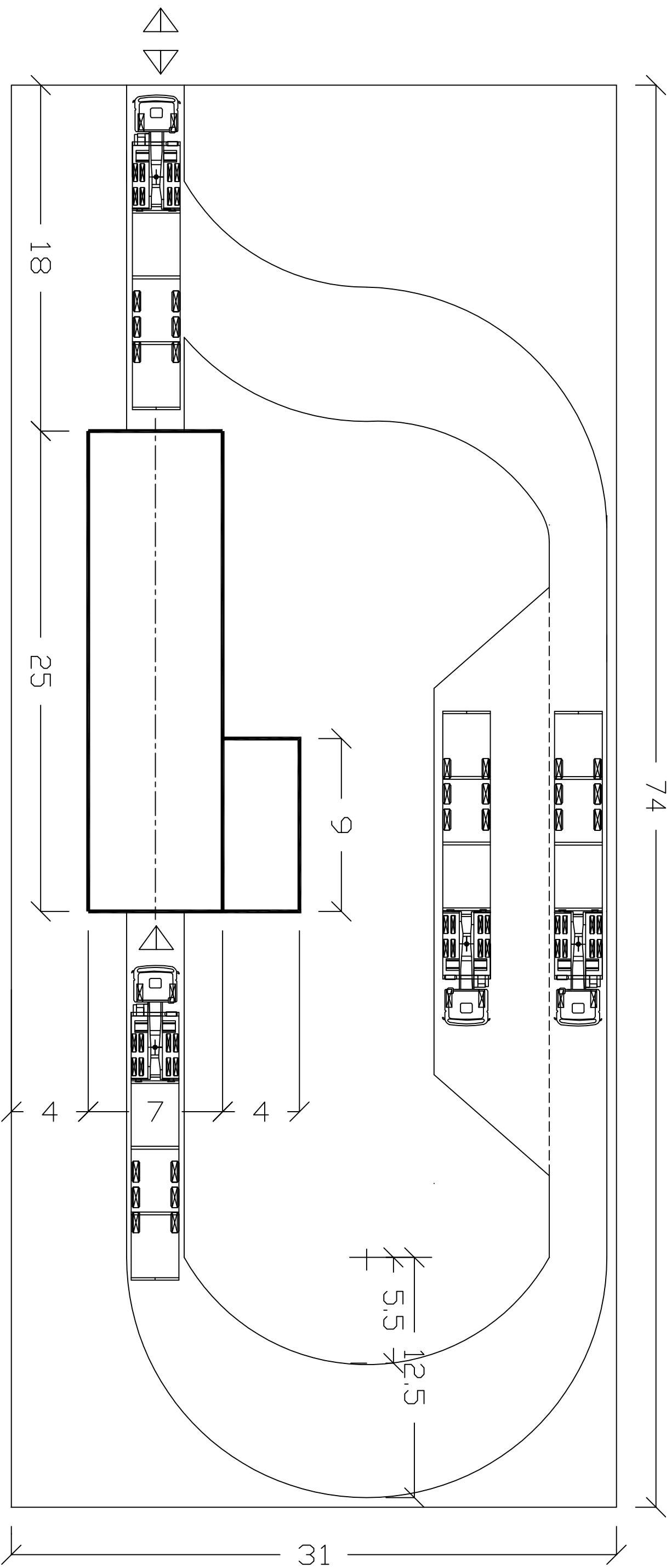
stacja kontroli pojazdów zagospodarowanie działki układ optymalny
